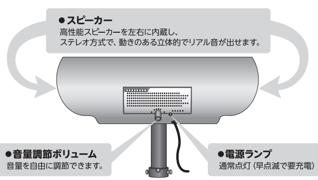
本体背面
